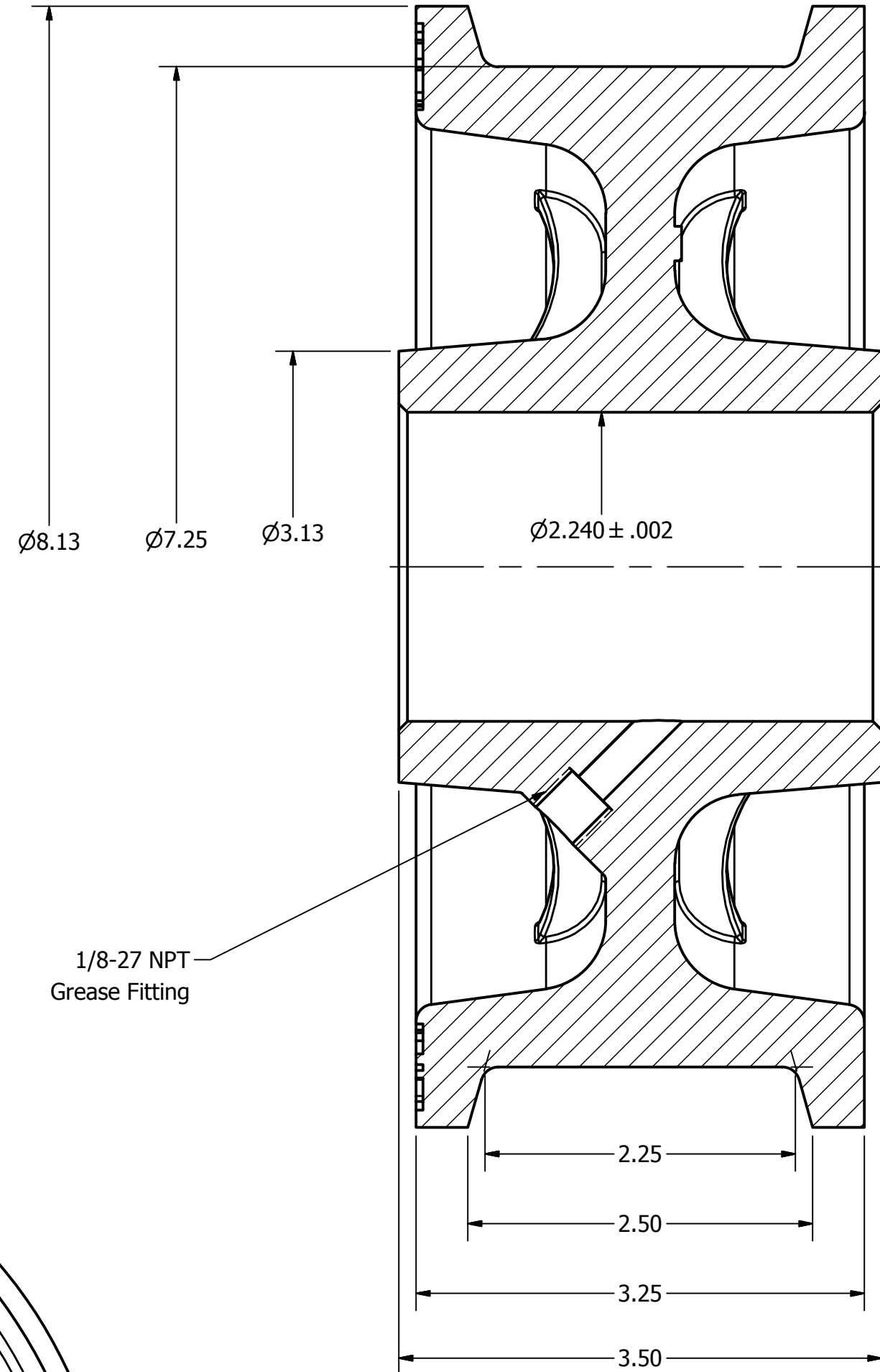
SECTION A-A
