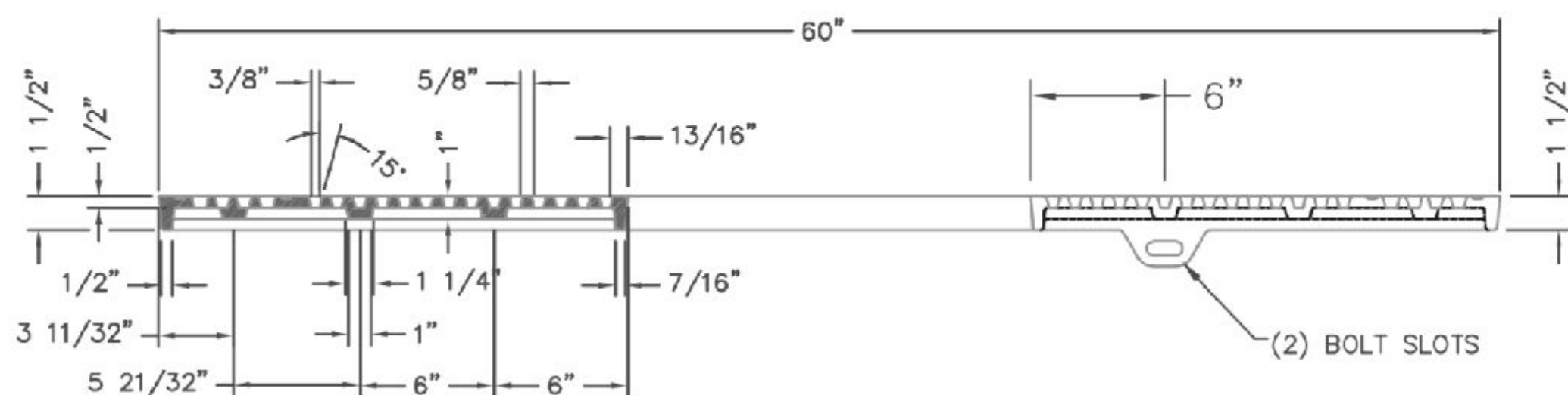
SECTION A-A
