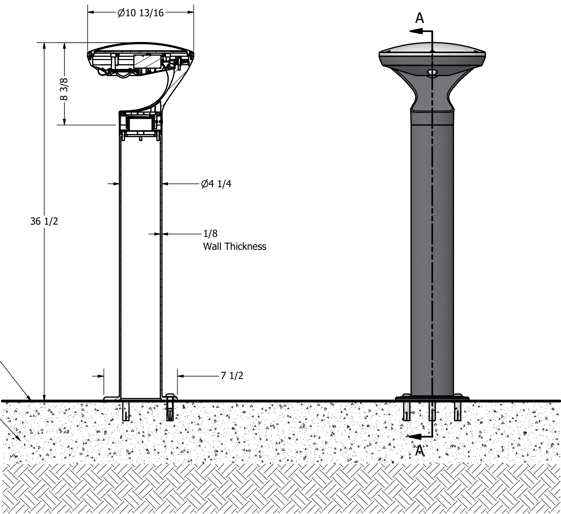
SECTION A-A
